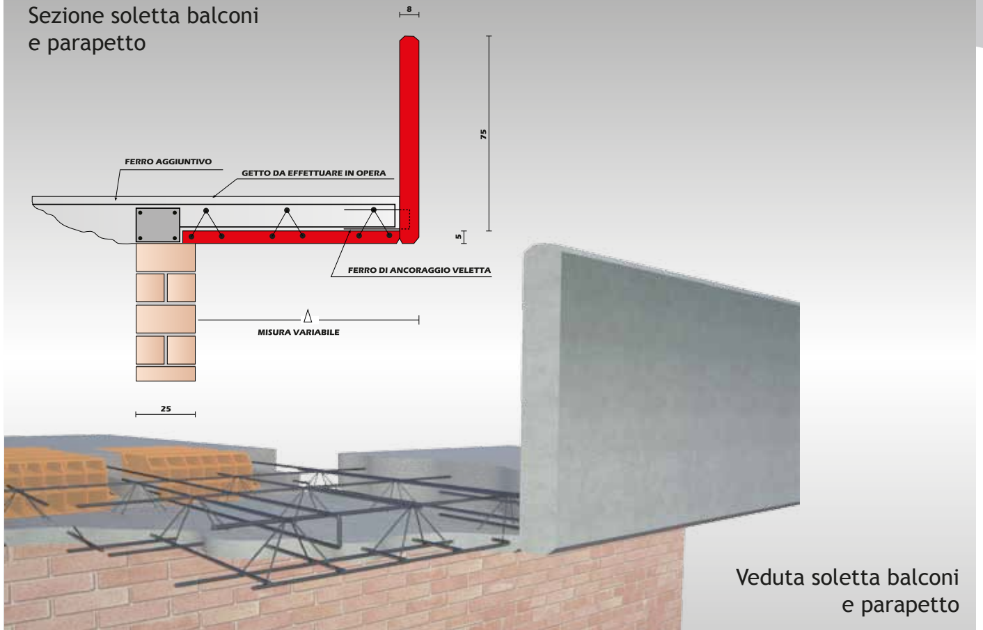
Sezione soletta balconi e parapetto sottosporgente
