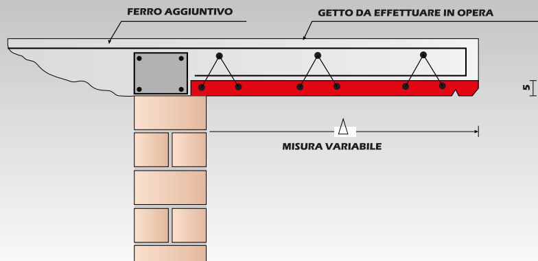
Sezione soletta balcone
