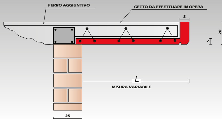
Sezione soletta balcone con testina
